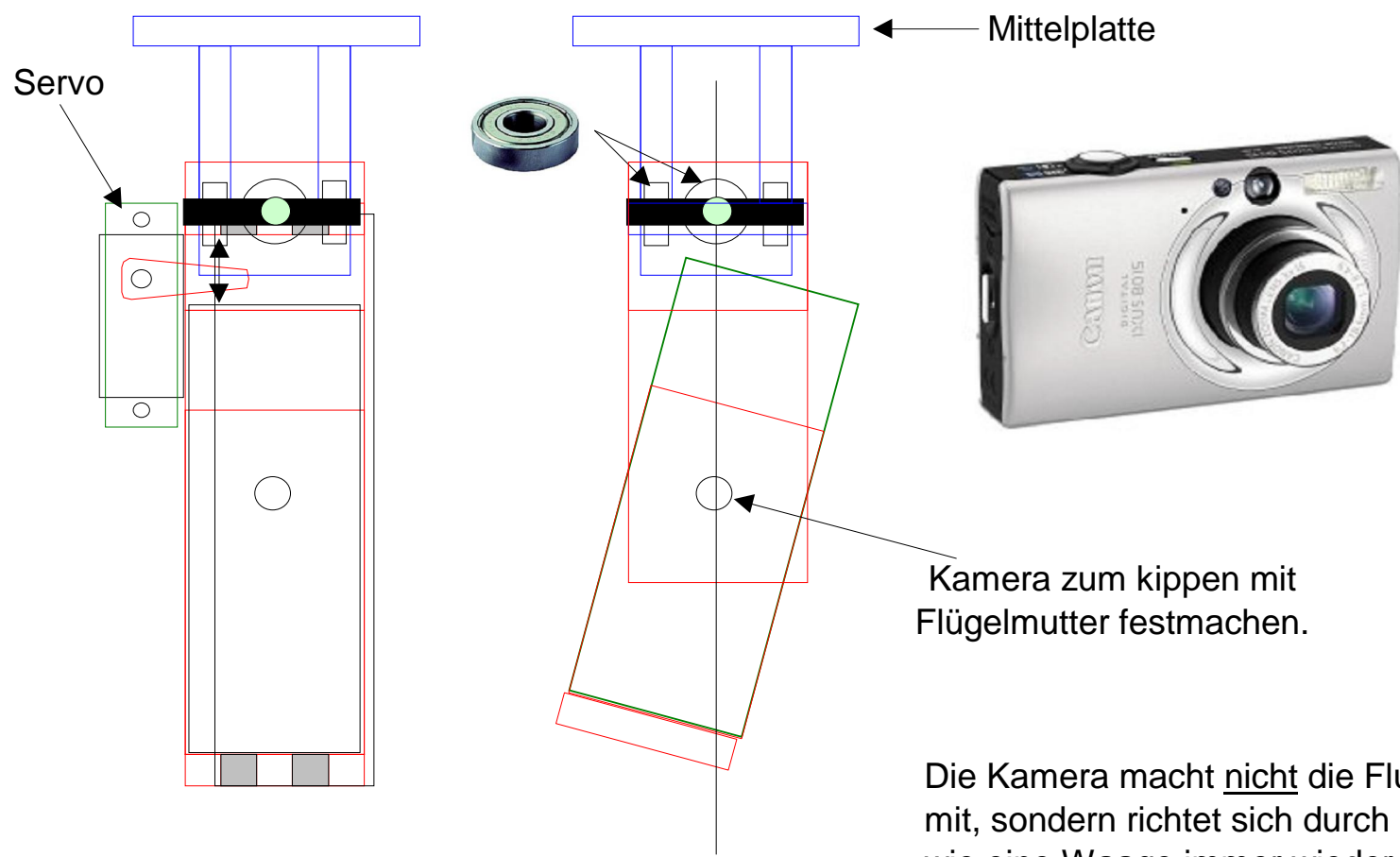
Seiten-Ansicht 1:1
